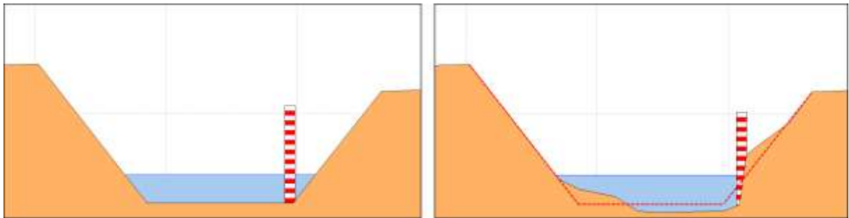
Figur 15-1 Ved en vandføringsevne forstås den mængde vand, vandløbet kan føre pr. tidsenhed ved en given vandspejlskote. Ovenstående principskitser viser, at vandføringsevnen (illustreret ved vandstanden) godt kan være til stede, selvom en del af tværsnitsarealet er fyldt op af aflejringer.
